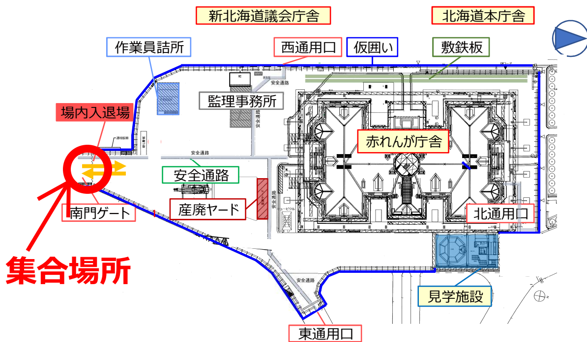
総合仮設計画図
